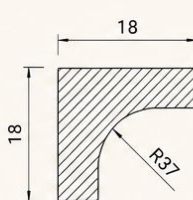
NỆP GÓC VUÔNG R37 2750*R37*18
