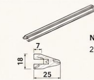
NỆP TRANG TRÍ 11 2750*25*18 (Có thể làm tay nắm)
