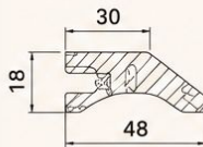
NỆP TRANG TRÍ 10 2750*48*18 (Có thể làm tay nắm)
