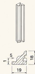
NỆP SÓNG Ồ VUÔNG
