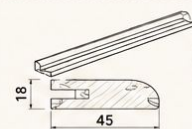
NỆP TRANG TRÍ 17 2750*45*18
