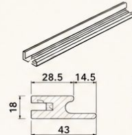
NỆP TRANG TRÍ 4 2750*43*18 (Có thể làm tay nắm)
