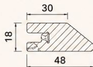
NỆP TRANG TRÍ 1 2750*48*18 (Có thể làm tay nắm)
