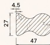
NỆP TRANG TRÍ 8 2750*47*27 (Có thể làm tay nắm)
