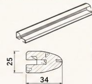
NỆP TRANG TRÍ 6 2750*34*25
