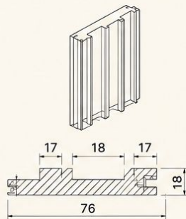
NỆP RÃNH DỌC
