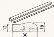
NỆP TRANG TRÍ 14 2750*30*18 (Có thể làm tay nắm)
