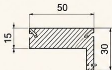
NỆP BỌC CỬA 2440/2745*50*30
