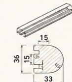
NỆP TRANG TRÍ 7 2750*33*36
