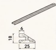
NỆP TRANG TRÍ 11 2750*25*18 (Có thể làm tay nắm)
