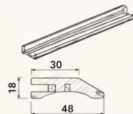
NỆP TRANG TRÍ 10 2750*48*18 (Có thể làm tay nắm)
