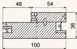
NỆP BỌC CỬA CHÍNH 2440/2745*100*36
