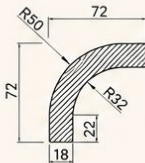
R50 – NỆP CONG R50
