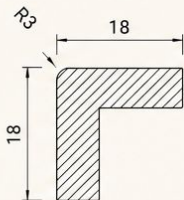
NỆP GÓC VUÔNG R3 2750*R3*18
