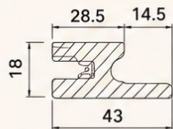
NỆP TRANG TRÍ 4 2750*43*18 (Có thể làm tay nắm)
