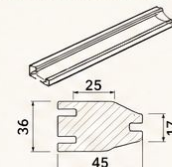
NỆP TRANG TRÍ 9 2750*45*36
