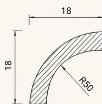
NỆP GÓC CONG R50 2750*R50*18
