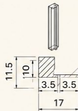
NỆP RÃNH DỌC
